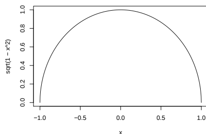
Rysunek 2: Wykres funkcji f(x) = \sqrt{1 - x^2}
