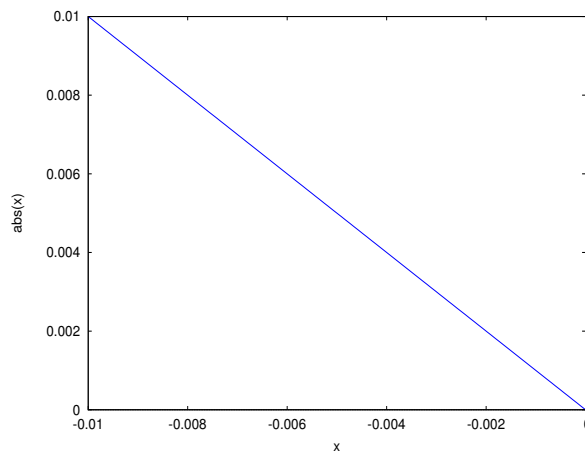
Rysunek 5: Wykres funkcji y = |x| na przedziale [-0,01; 0]
