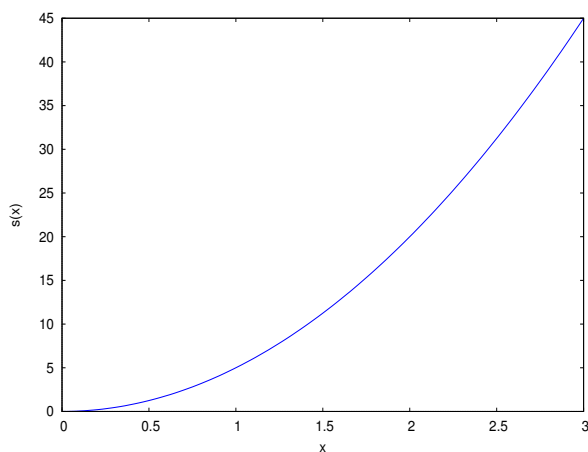
Rysunek 1: Wykres funkcji s na przedziale [0, 3]
