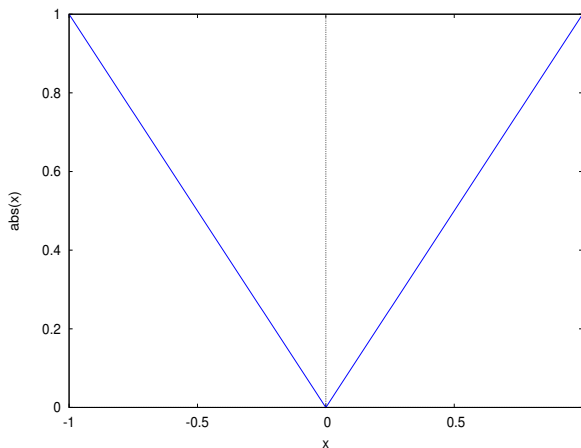
Rysunek 4: Wykres funkcji y = |x| na przedziale [-1; 1]
